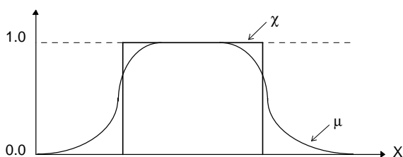
FIGURA 1 - Função característica \chi , para um conjunto clássico e função de pertinência \mu , para um conjunto fuzzy (adaptado de Hu et al. , 1996).
